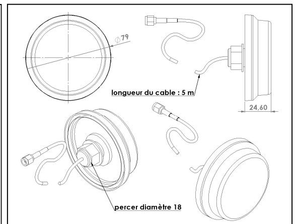
Antenne déportée 3G
